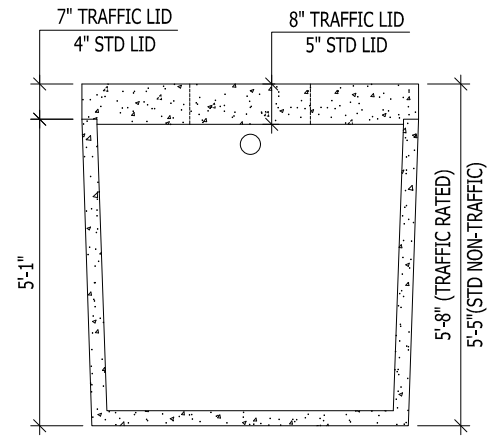
SECTION B SCALE: NTS
