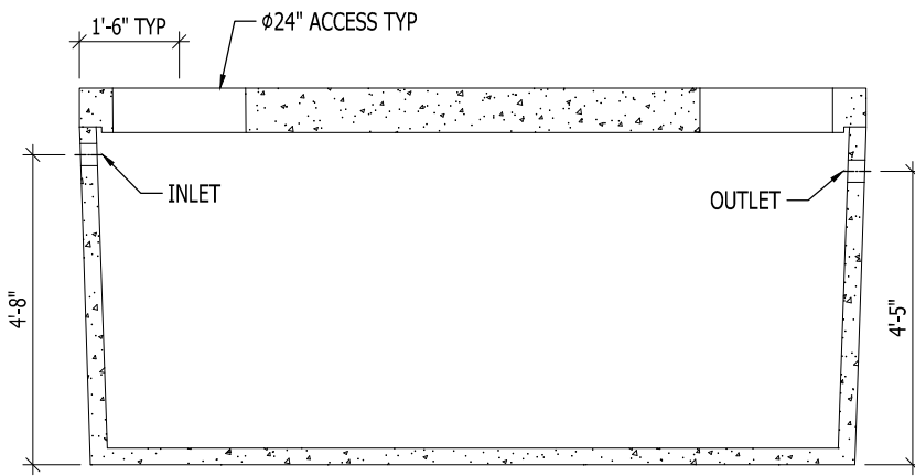
SECTION A SCALE: NTS
